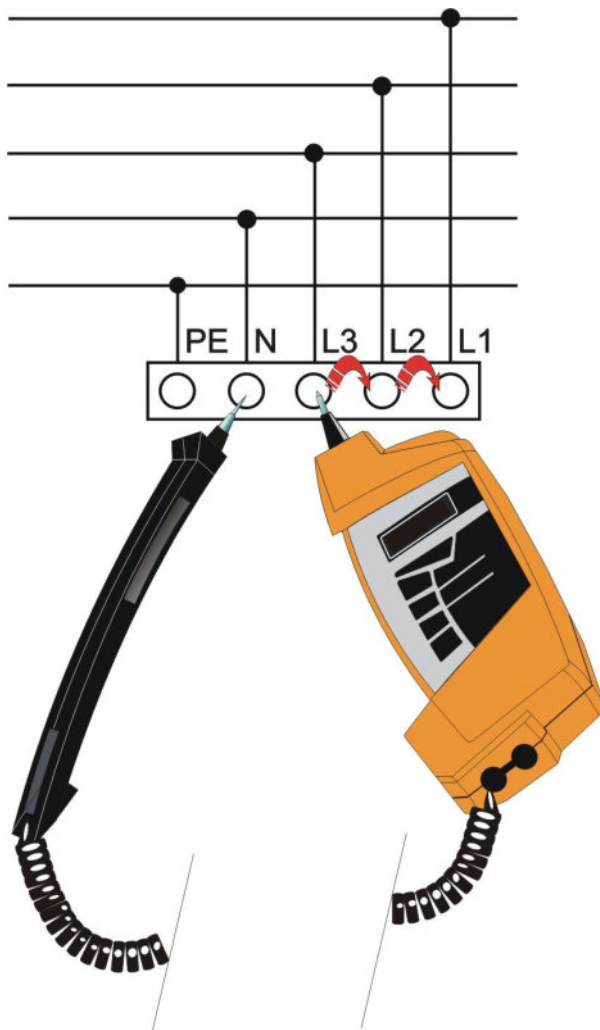
Obr. 3.3 Příklad zapojení
