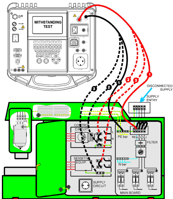
Obr. 2 – Zkouška izolací přiložením výdržného napětí průmyslového kmitočtu
