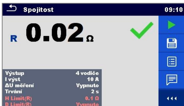
Obr. 6 – Ověření spojitosti PE obvodu
