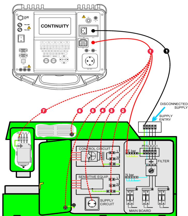
Obr. 1 – Měření spojitosti PE obvodu
