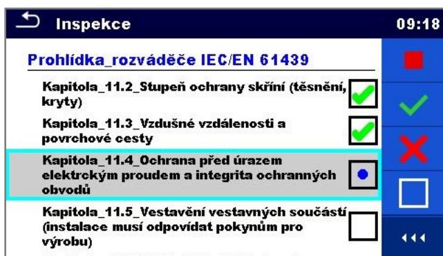
Obr. 4 – Výsledky prohlídky rozvaděče
