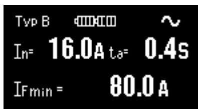
Obr. 3.16. Zobrazení min. zkratového proudu nutného pro vybavení ochrany
